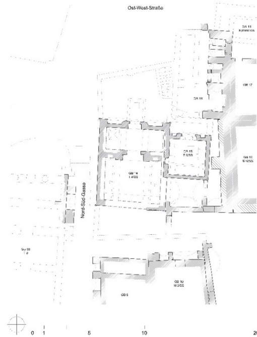
Tuna el-Gebel, Petosiris-Nekropole Grundriss GB 14-15 - ohne Maßstab -
